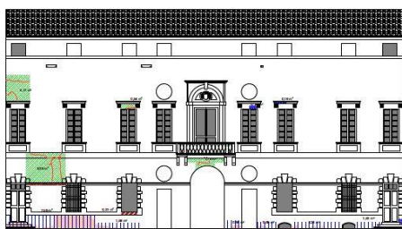
Prospetto A-A
